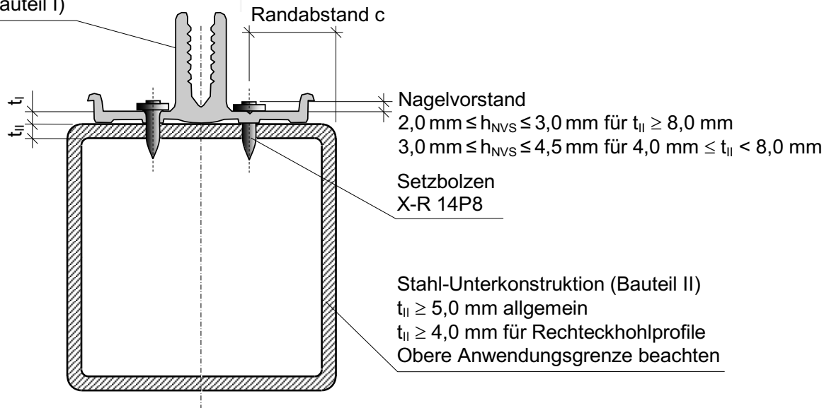
MBJ Aluminium-Aufsatzprofil Art.-Nr. 2520 / 2520-B (Bauteil I)
