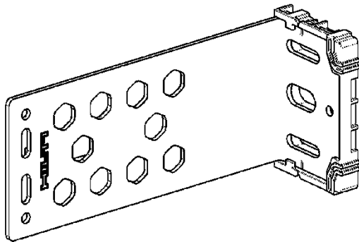
Konsole MFT-VS M Konsole MFT-VSI M**
