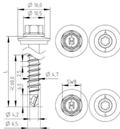
Hilti S-MDW 51 S 6,5xL * (Typ M2) Hilti S-MDW 51 SS 6,5xL ** (Typ M2)
