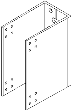
Konsole MFT-S2S U L / MFT-S2S UI L*
