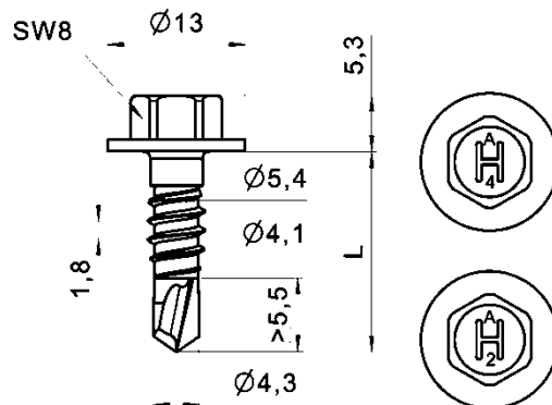
Hilti S-AD 01 S 5,5xL * (Typ G) Hilti S-AD 01 SS 5,5xL ** (Typ G)
