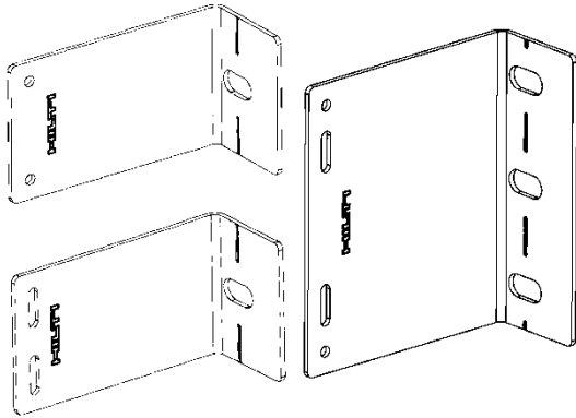
Konsole MFT-FOX VTR SP M 11 / MFT-FOX VTR FP M 11 Konsole MFT-FOX VTR L 11
