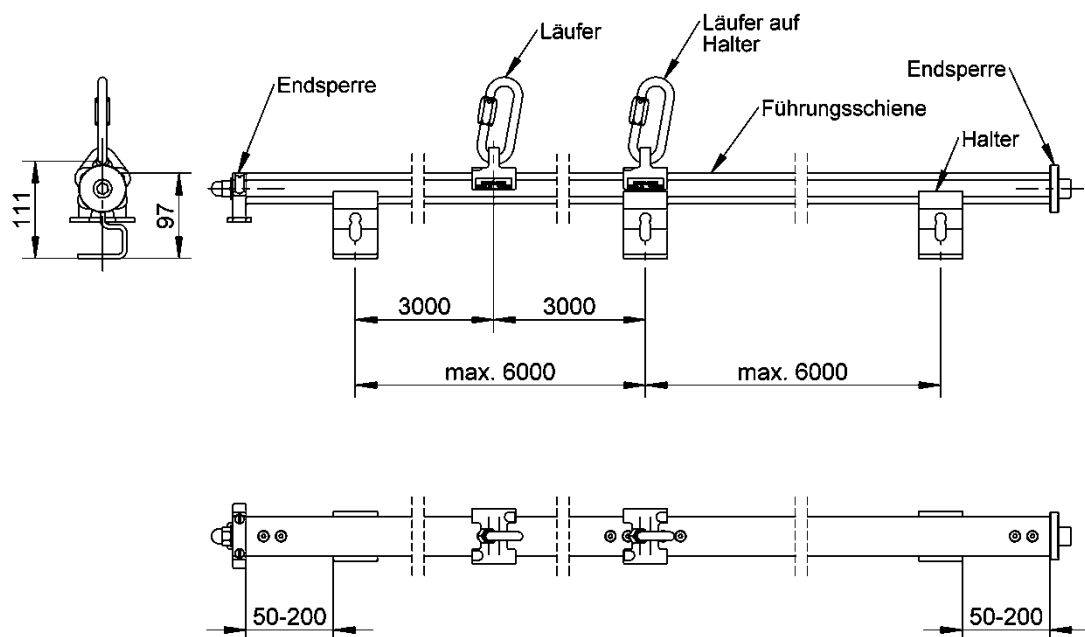
Abbildung 1 - Lasteinleitung in den Baukörper [Maße in mm]
