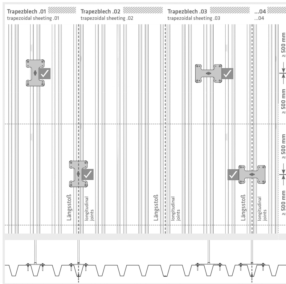
Abbildung 1 - Montagevorgaben auf Trapezprofil bei Absturzrichtung in Trapezprofilspannrichtung
