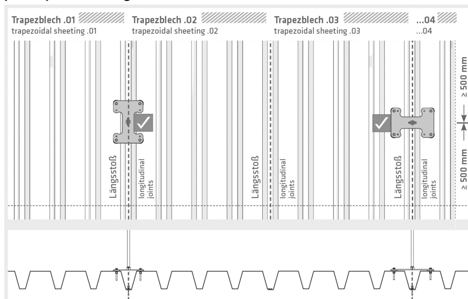
Abbildung 2 - Montagevorgaben auf Trapezprofil bei Absturzrichtung quer zur Trapezprofilspannrichtung
