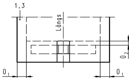
EN 1337-1, Nr. 1.2 Elastomerlager mit Führungslager
