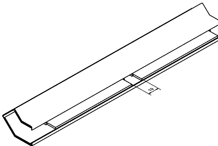
135°- Abdeckblech (Ausführungsbeispiel)
