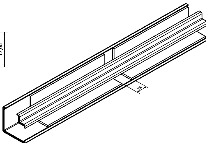
90°- Abdeckblech (Ausführungsbeispiel)
