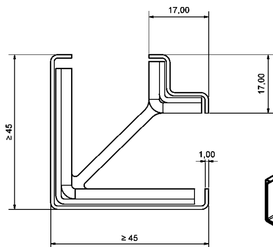
90°- Abdeckblech (Ausführungsbeispiel)
