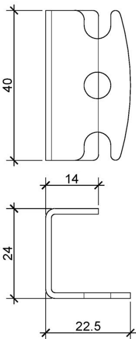
▲ Glashalter seitlich, Var. 1.2 ZHC2720-LR40-0015
