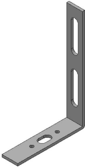
▲ Ständer-Befestigungswinkel, Var. 3 ZSR2135, Abm. 130x85x20x3 ZBV2102, Abm. 105x66x56x1
