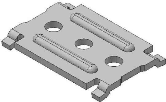
▲ Befestigungsbügel ZUV2137, Abm. 38x56x7,5 ZUV2138, Abm. 81x56x7,5
