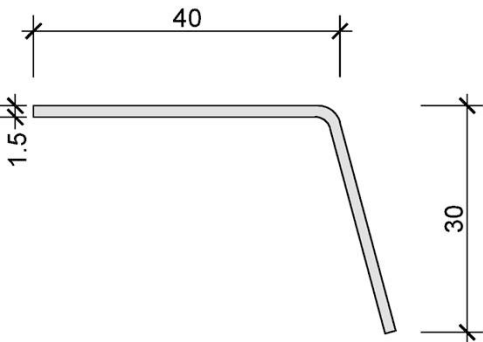
▲ Wandanschluss- Winkelprofil Abm. 40x30x1,5
