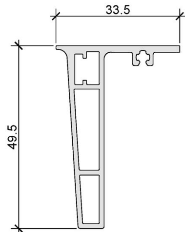
▲ Verglasungsprofil 50 AV-2737, Glas 6, Typ I
