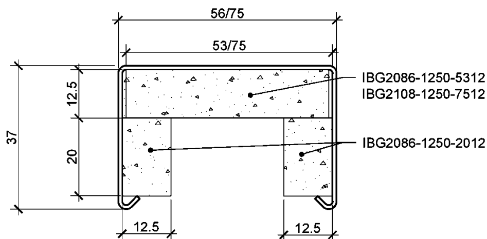
▲ Querkämpfer
