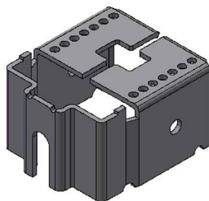
▲ Querkämpferwinkel ZQV2086-0000-0020
