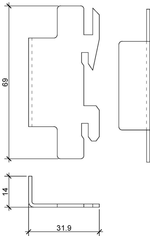
▲ Glashalter seitlich, Var. 1.1 ZHC2720-L/R069-0015
