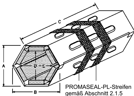
"FST Kabelbox Kombi R6+" für den Einbau mit Bauschaum
