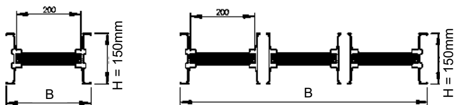
Stromschiene (Ausrichtung der Leitschienen „horizontal“)
