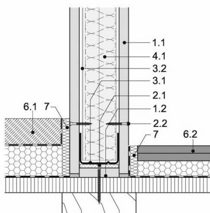
Anschluss Holzbalkendecke (Systemskizze)
