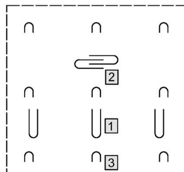
Unterkante Tragschicht
