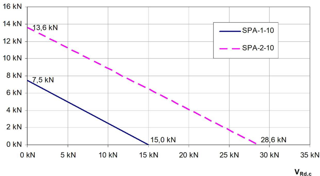
Diagr. 5: Betontragfähigkeitslinie SPA-10
