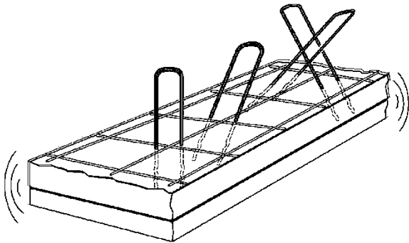
Bild 18: Nachverdichten der unteren Schicht (SPA-N, SPA-FLEX). Einhalten der Ankerlänge im Beton gemäß Anlagen 5 und 6.
