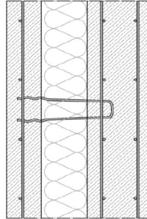
Verbundnadel SPA-N
