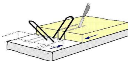
Bild 15: Einbau Wärmedämmung SPA-2
