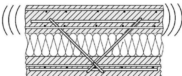
Bild 20: Betonieren und Verdichten der oberen Schicht
