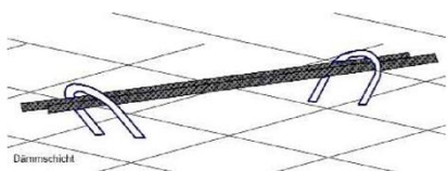
Bild 2: Tragschicht
