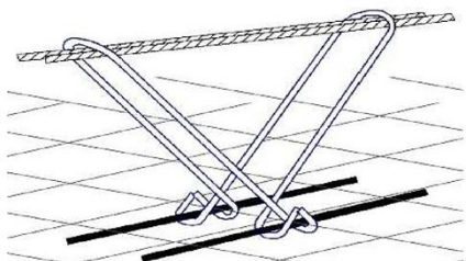
Bild 1: Vorsatzschicht
