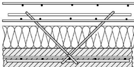
Bild 19: Einbau der Bewehrung der oberen Schicht
