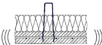
Bild 12: Einbau SPA-N und nachverdichten
