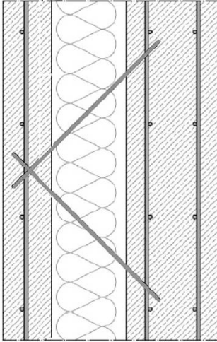
Stabtraganker SPA-1/ -2
