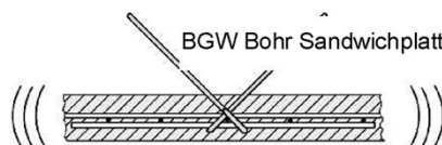
Bild 13: Verdichten des Betons
