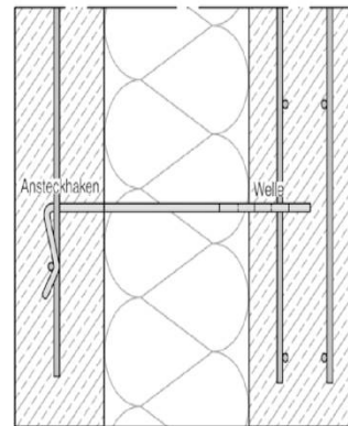
Anstecknadel SPA-A
