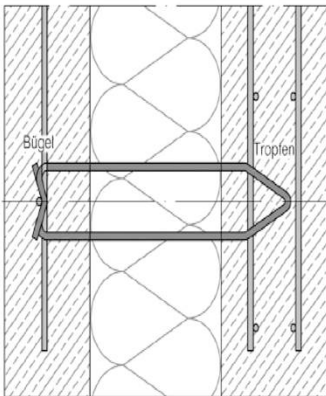
Verbundbügel SPA-B
