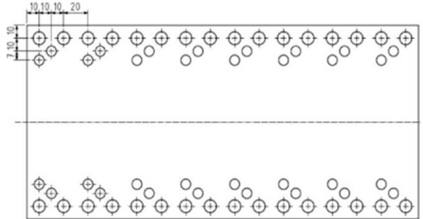
Manschettenankerblech in der Abwicklung
