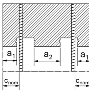
b) mehrteilig (zwei zweireihige Anschlüsse)
