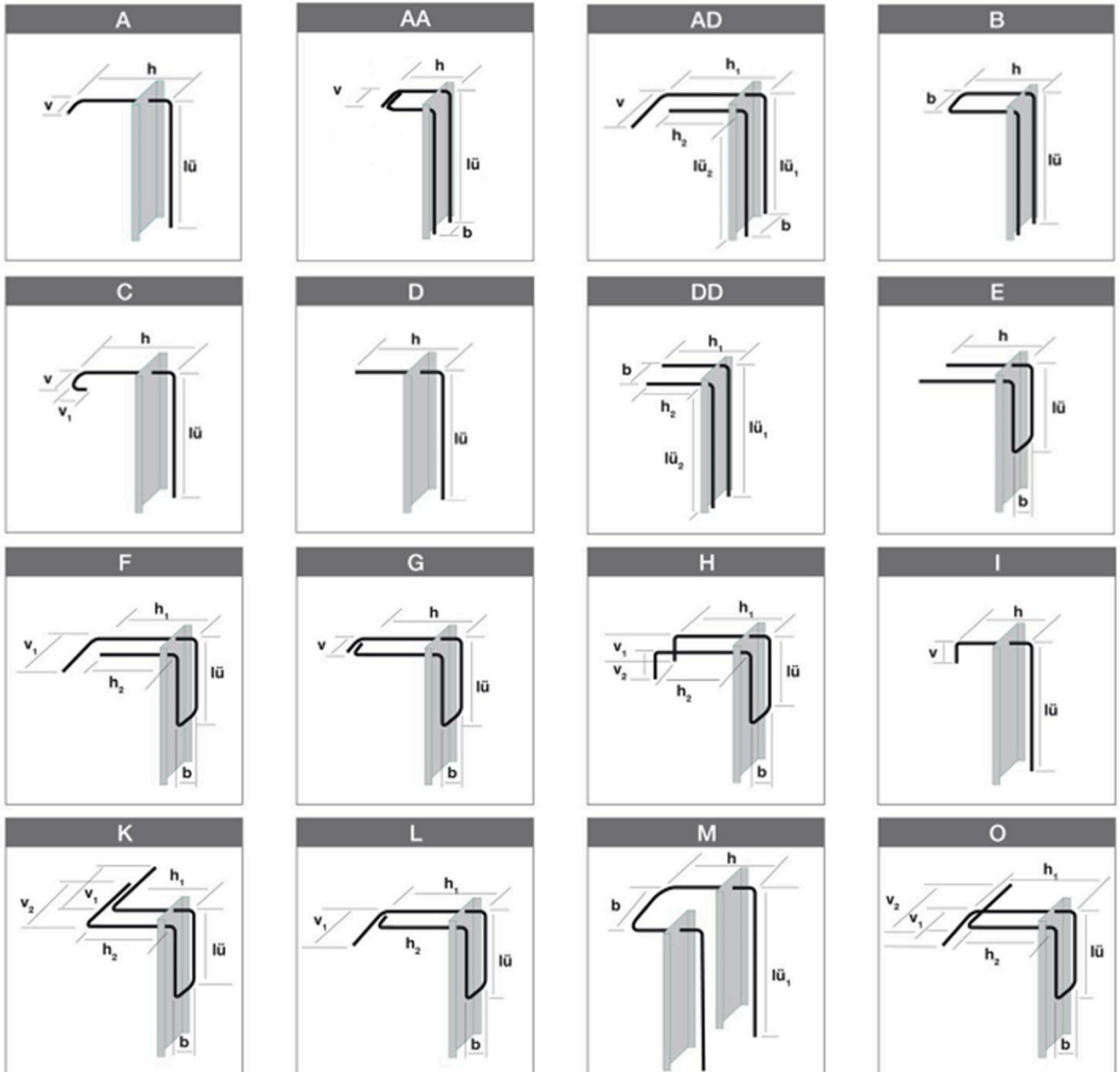
Abbildung 5: Biegeformen der Rückbiegebewehrung, Beispiele
