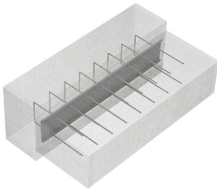
a) Decke – Wand
