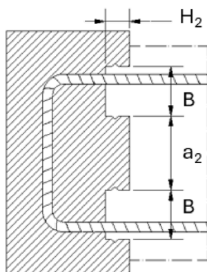
Abbildung 8: Verzahnte Fugenausbildung nach DIN EN 1992-1-1, Bild 6.9
