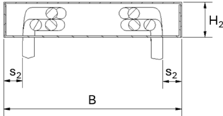
Abbildung 4: Querschnitt Verwahrkasten und Deckel
