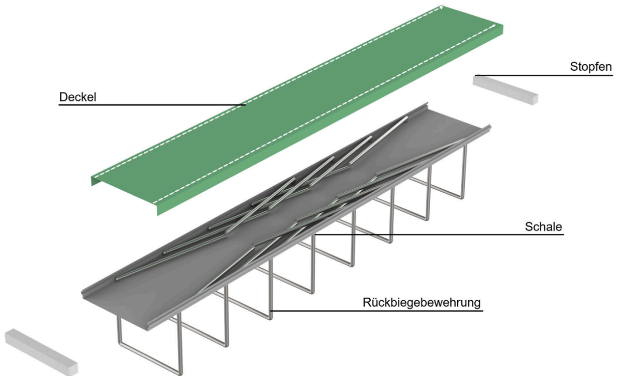
Abbildung 3: Aufbau zweireihiger Rückbiegeanschluss
