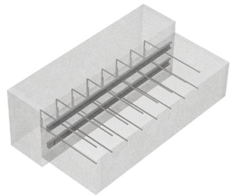
b) Podest – Wand
