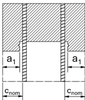
a) einteilig (zweireihiger Anschluss)
