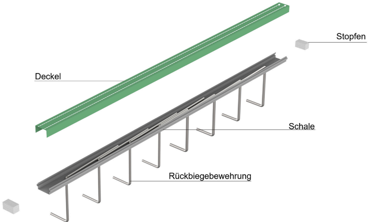
Abbildung 2: Aufbau einreihiger Rückbiegeanschluss
