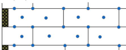
9 (5/4) Dübel/m 2
