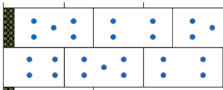
9 Dübel/ m 2
