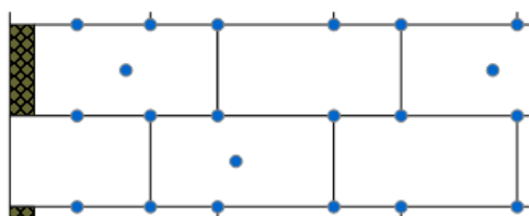
5 (1/4) Dübel/m 2
