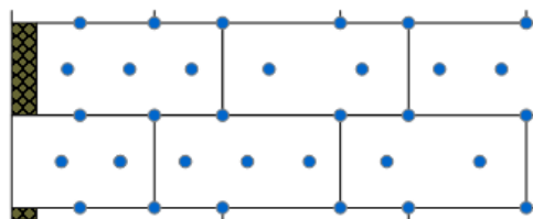
9 (5/4) Dübel/m 2
