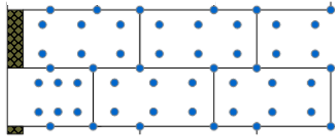
16 (12/4) Dübel/m 2
