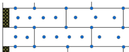
11 (7/4) Dübel/m 2
