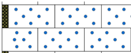
16 Dübel/ m 2
