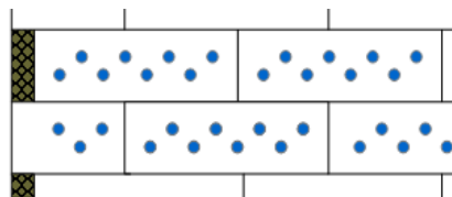
16 Befestigungsmittel/m 2
