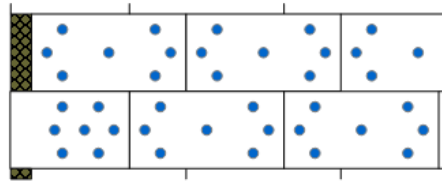
16 Befestigungsmittel/m 2
