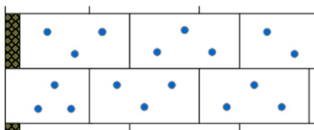
7 Befestigungsmittel/m 2
