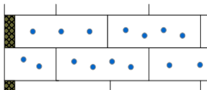
8 Befestigungsmittel/m 2
