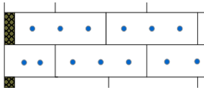
7 Befestigungsmittel/m 2
