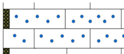
12 Befestigungsmittel/m 2
