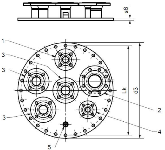
Domdeckel mit Flanschanschlüssen
