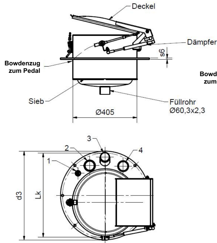
Domdeckel DN500 mit Einfülltrichter
