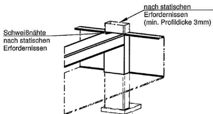
Anbindung Mittelrahmen
