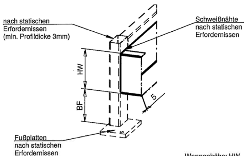
Anbindung Außenrahmen
