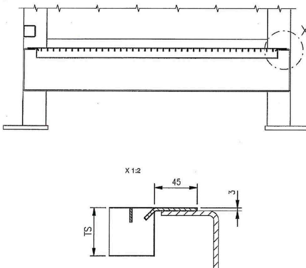
Einbaudetail Gitterroste
