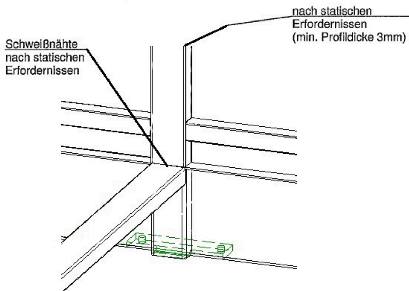
Anbindung Mittelrahmen
