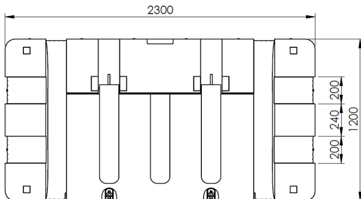
Draufsicht
