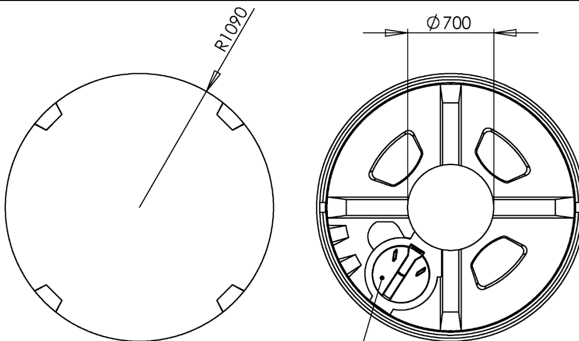
Grundriss
