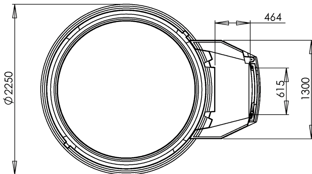
Grundriss
