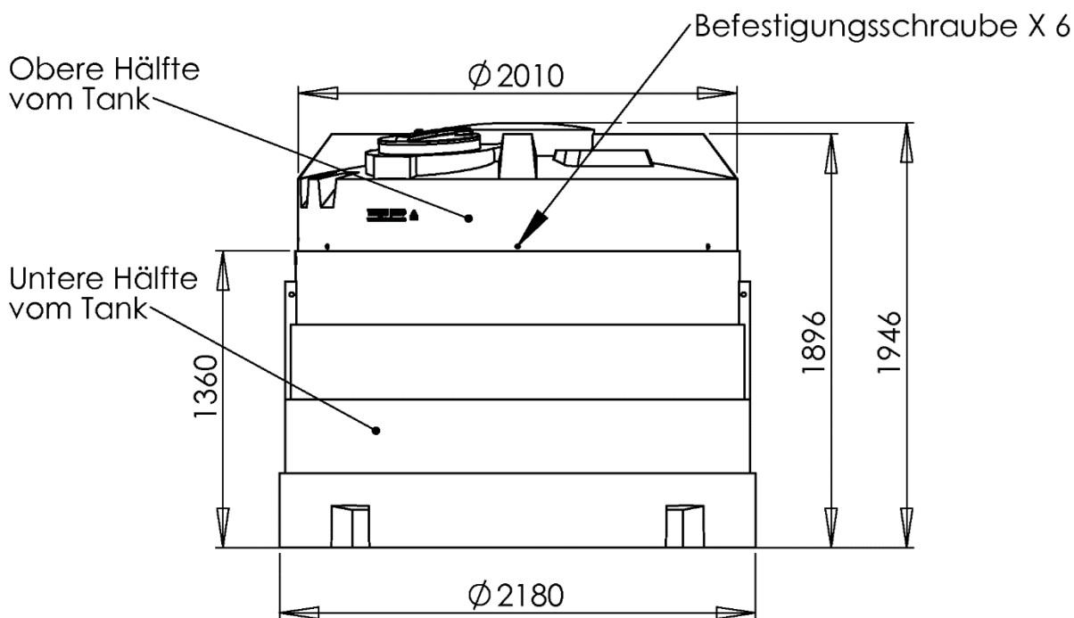
Seitenansicht
