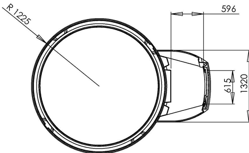
Grundriss
