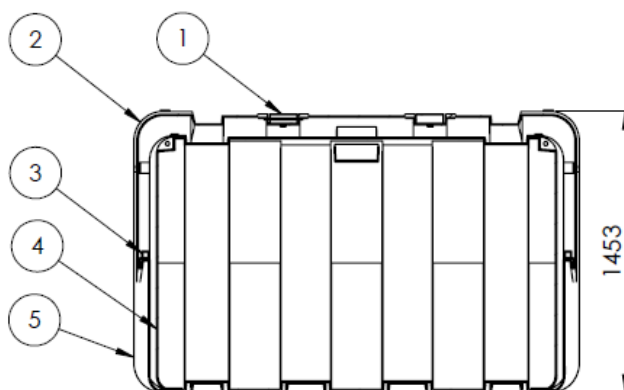
SCHNITT A-A
