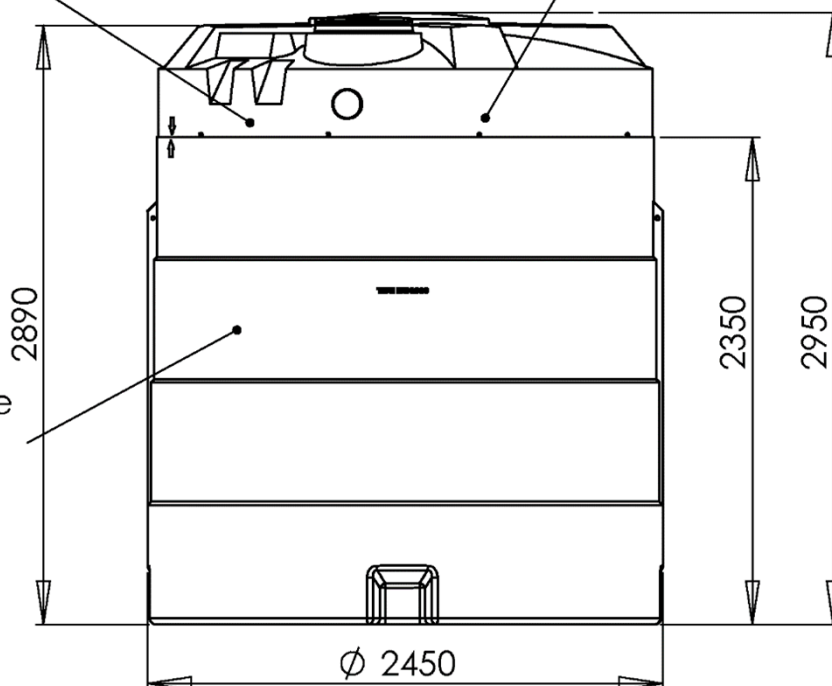
Seitenansicht
