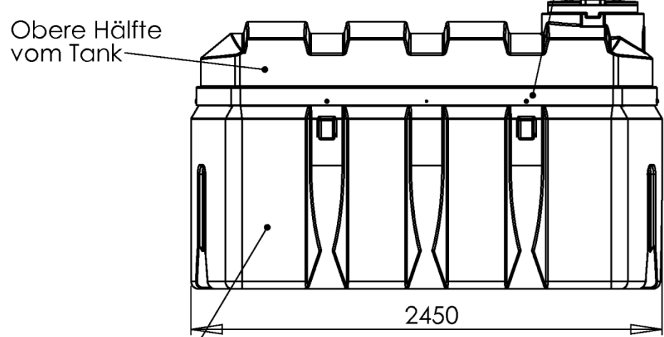
Seitenansicht
