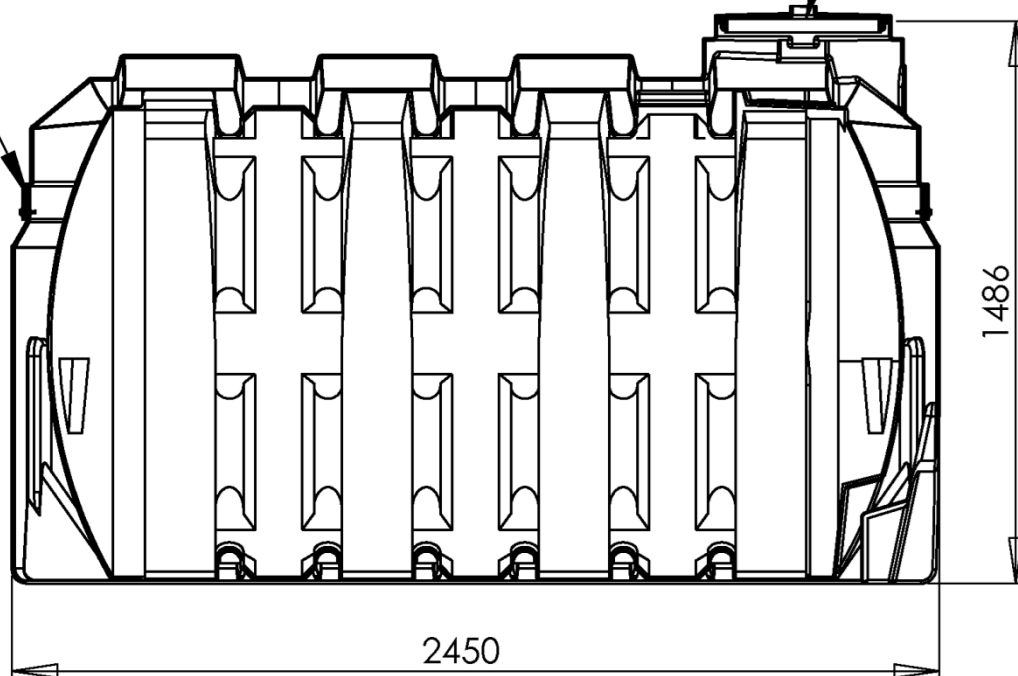
Grundriss
