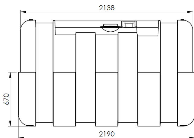
Vorderansicht
