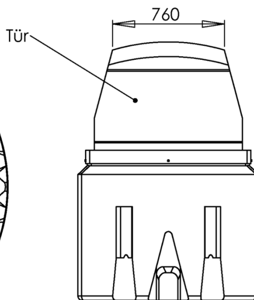
Vorderansicht
