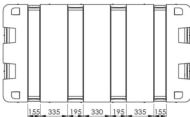
Untersicht
