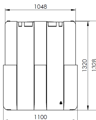
Seitenansicht
