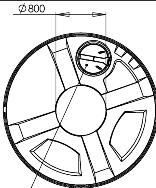
Obere Draufsicht
