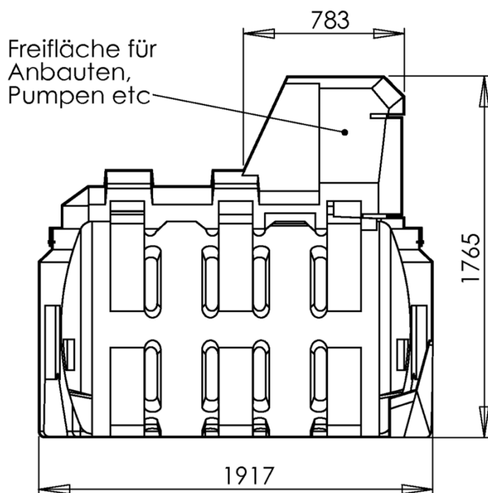
Seitenansicht - Querschnitt
