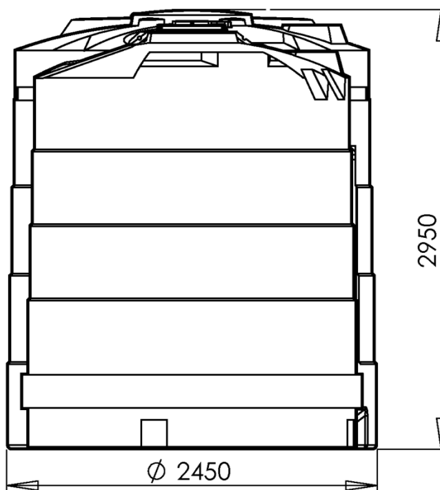
Seitenansicht - Querschnitt
