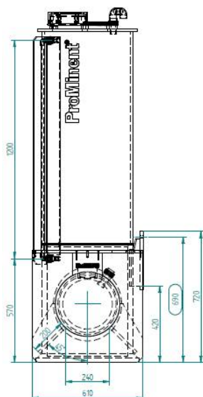
Innenbehälter 200 I
