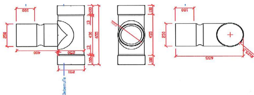
202.723A Klebe-T-Stück Ø250 Typ 40cm
