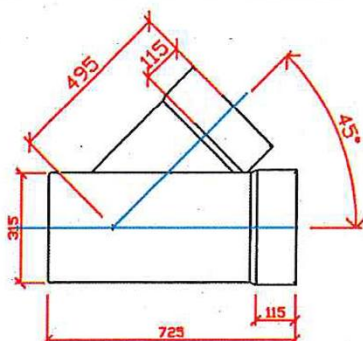
202.749 Klebeabzweiger 300/300 45° 2 Muffe Grau
