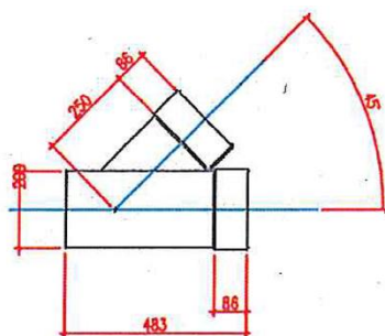
202.747 Klebeabzweiger 200/200 45° 2 Muffe Grau
