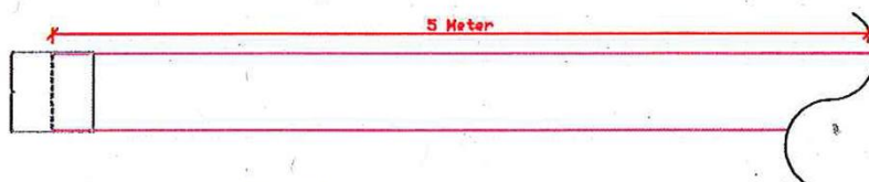
191.048 KG Rohr Ø200mm *5m (mit Doppelter Klebemuffe)
