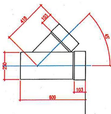
202.748 Klebeabzweiger 250/250 45° 2 Muffe Grau
