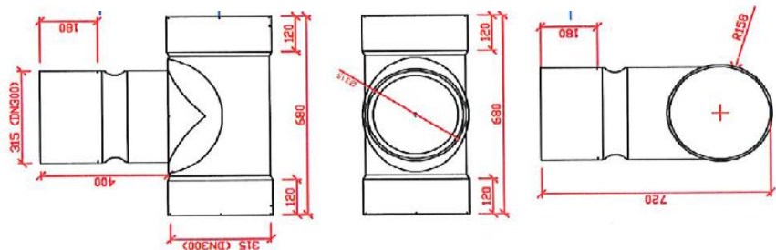
202.724A Klebe-T-Stück Ø300 90° Typ 40cm
