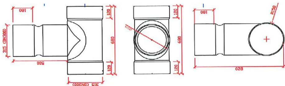
202.724B Klebe-T-Stück Ø300 90° Typ 50cm
