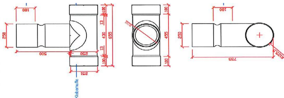
202.723B Klebe-T-Stück Ø250 Typ 50cm
