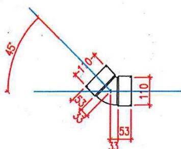
202.740 Bogen Grau Ø110 45° 2 Klebemuffen
