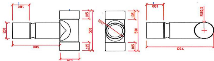
202.722B Klebe-T-Stück Ø200 90° Typ 50cm
