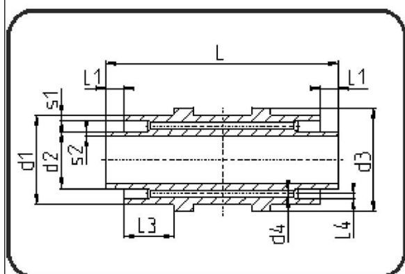
Poly-Flo Festpunkt mit Schulter und Cut Out
