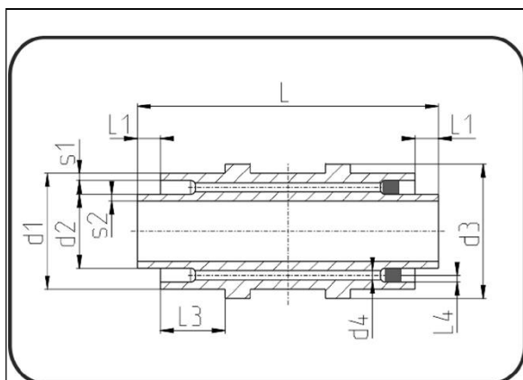
Poly-Flo Festpunkt mit Schulter ohne Cut Out
