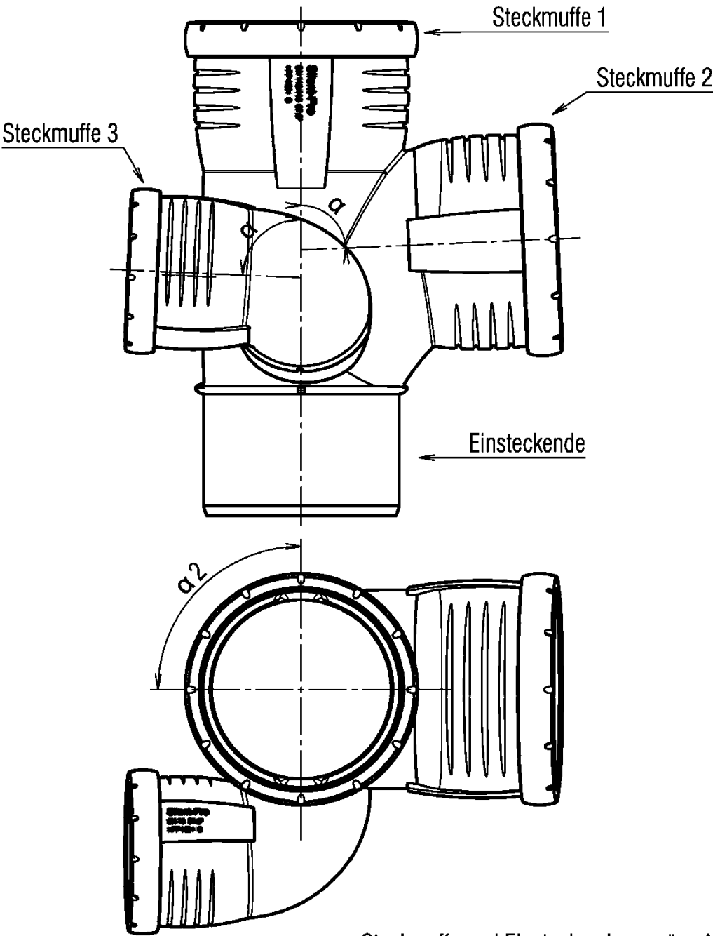
Steckmuffe und Einsteckende gemäss Anlage 4
