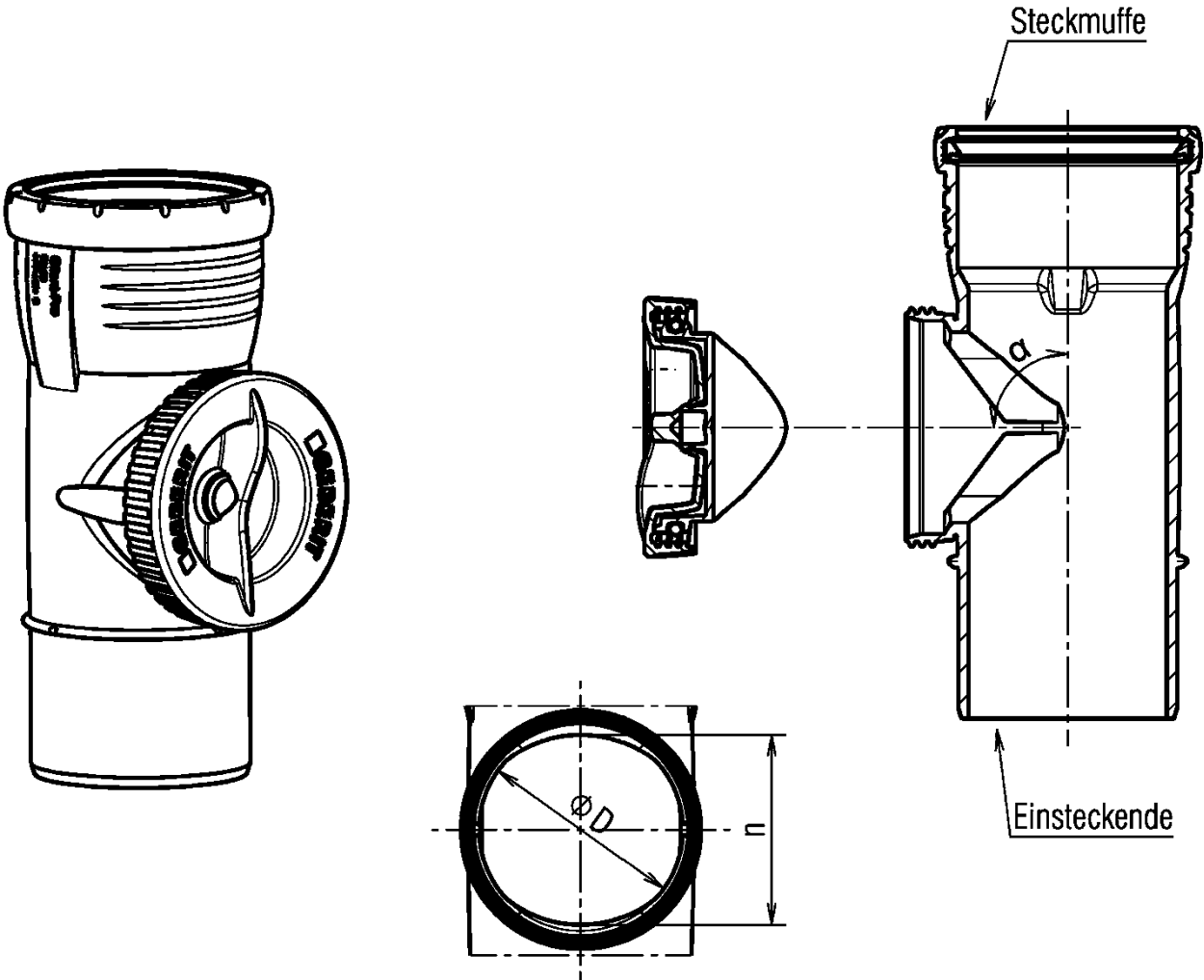
Steckmuffe und Einsteckende gemäss Anlage 4
