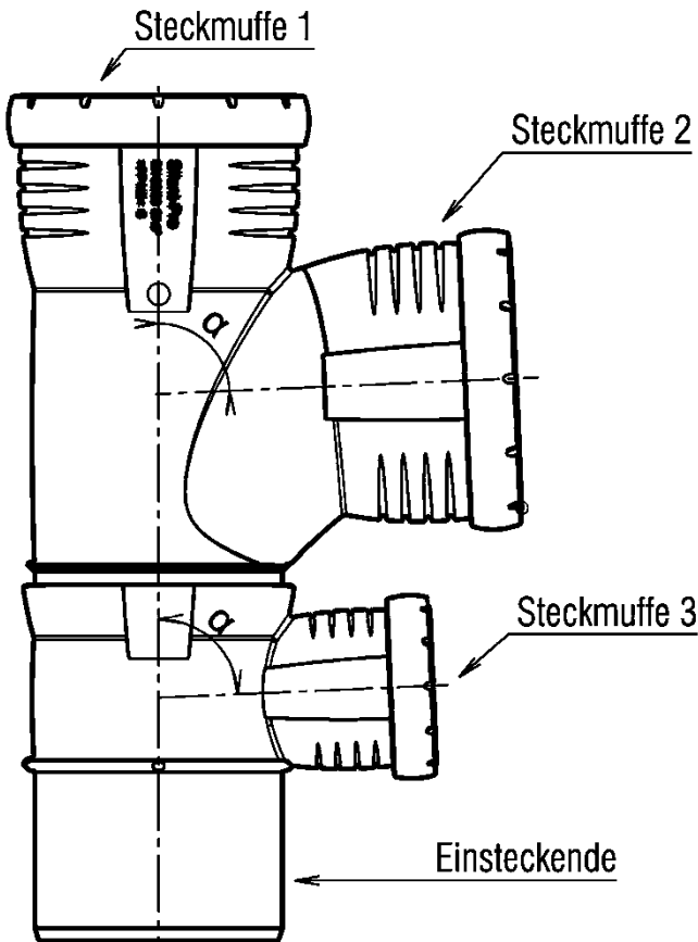
Steckmuffe gemäss Anlage 4
