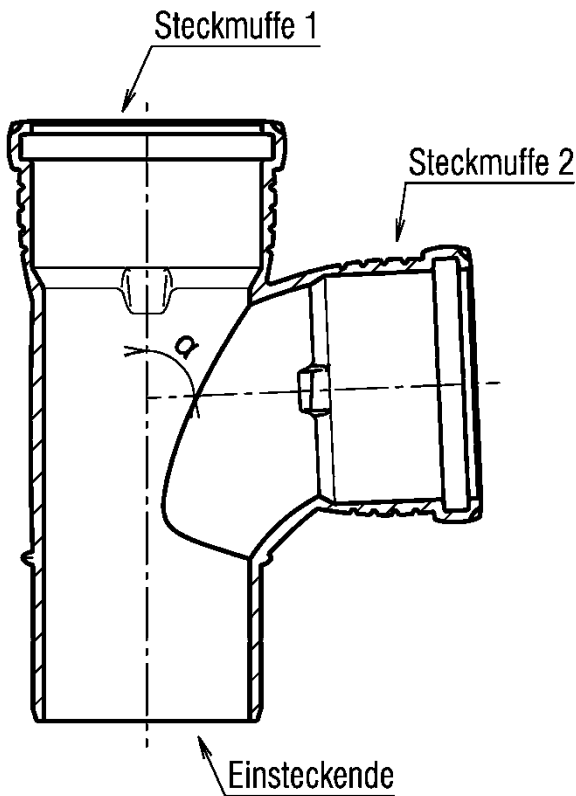
Steckmuffen und Einsteckende gemäss Anlage 4
