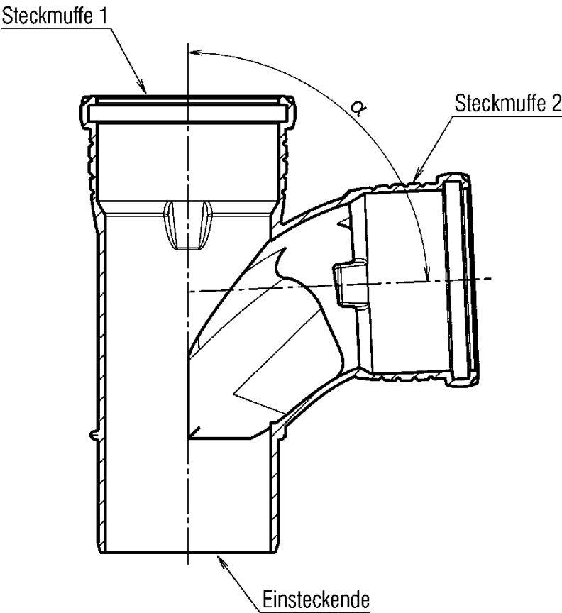
Steckmuffen und Einsteckende gemäss Anlage 4
