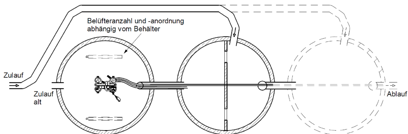
Grobfang Schlamm-speicher
