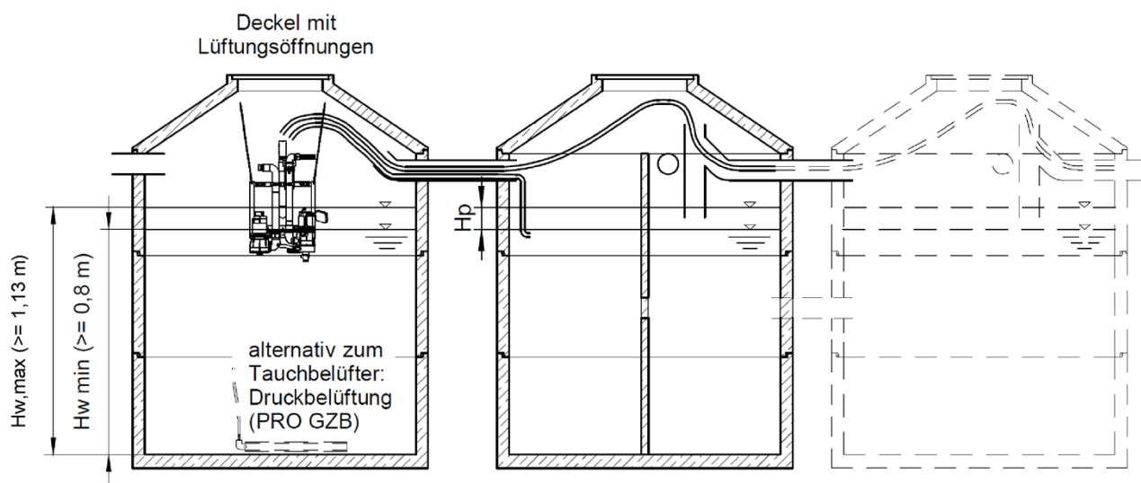
Grobfang Schlamm-speicher
