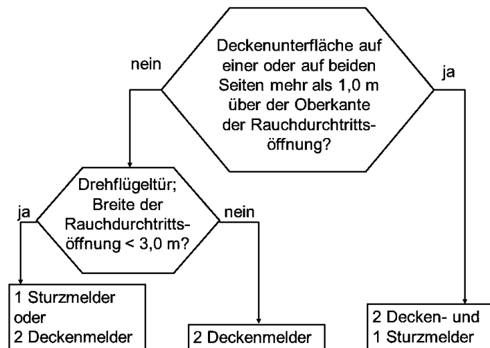
Bild 4: Entscheidungsdiagramm
