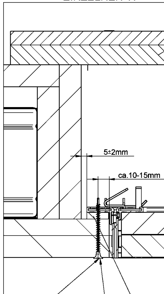
EINZELHEIT K
