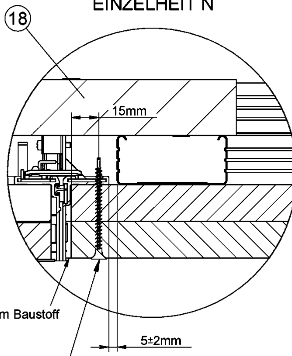
EINZELHEIT N
