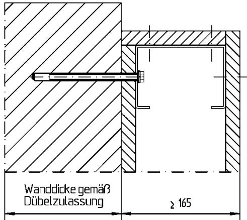
wahlweise Wandbefestigung
