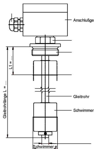
Schwimmer Magnetschalter Typ:A... und Typ:60...
