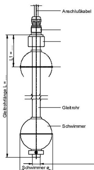
Schwimmer Magnetschalter Typ:E...
