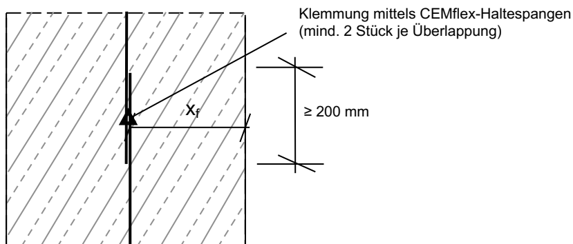
Abbildung 3: Verbindung der Fugenbleche durch Überlappung und Klemmung
