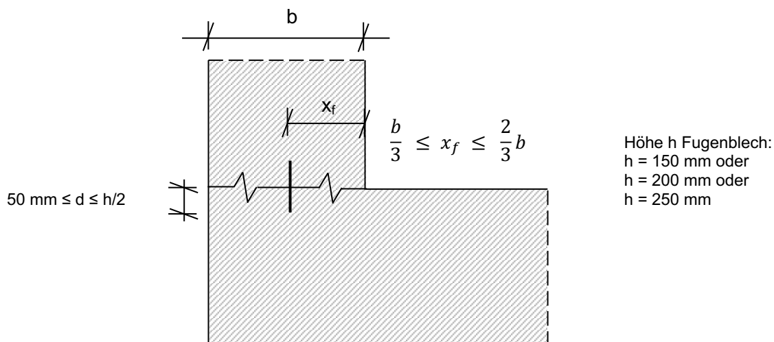
Abbildung 1: Schematische Darstellung Einbautiefe d des Fugenblechs
