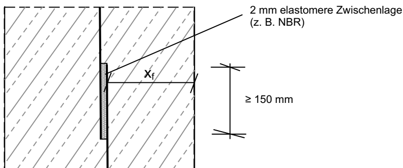
Abbildung 1: Verbindung der Fugenbleche durch Klemmen mit elastomerer Zwischenlage gemäß DAfStb-Richtlinie "BUMwS"
