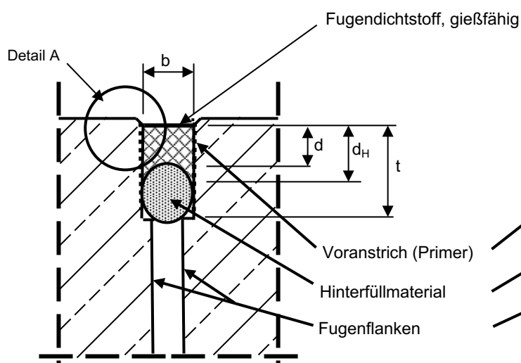
befahrbare Fugenkonstruktion
