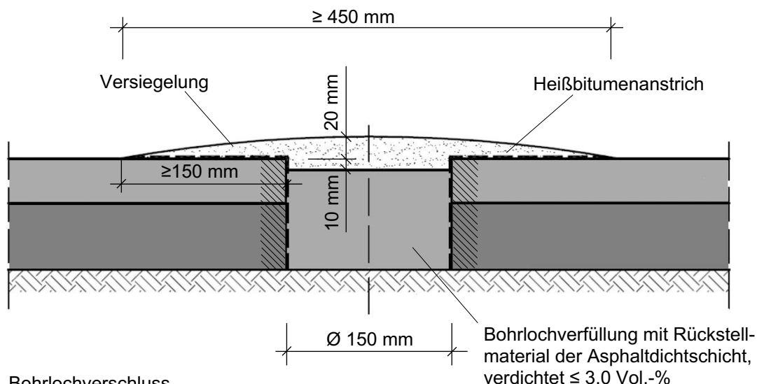
Bild 1: Bohrlochverschluss
