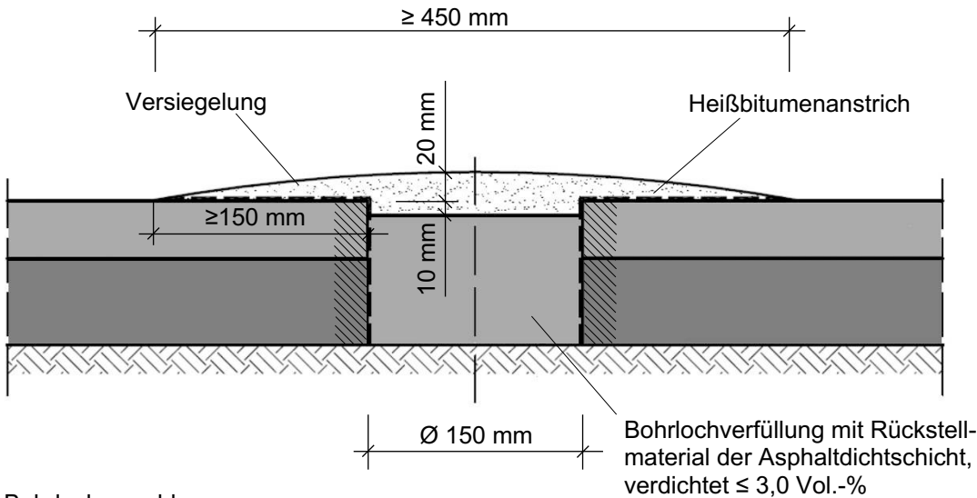
Bild 1: Bohrlochverschluss
