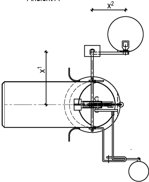
Ansicht A
