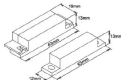
Magnetkontakt
