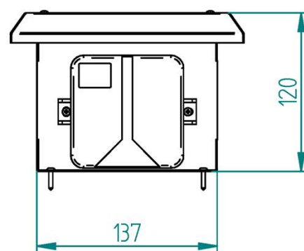
Ansicht von vorn
