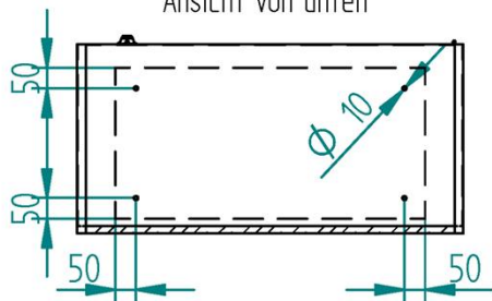
FSE-30 F Ansicht von unten
