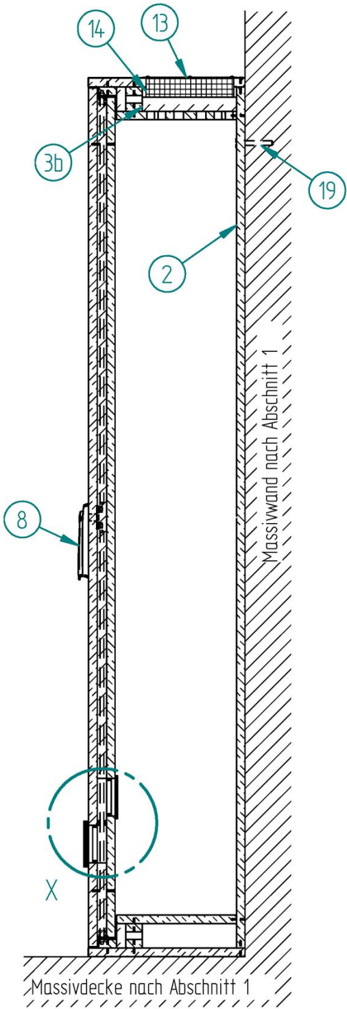
Schnitt B-B
