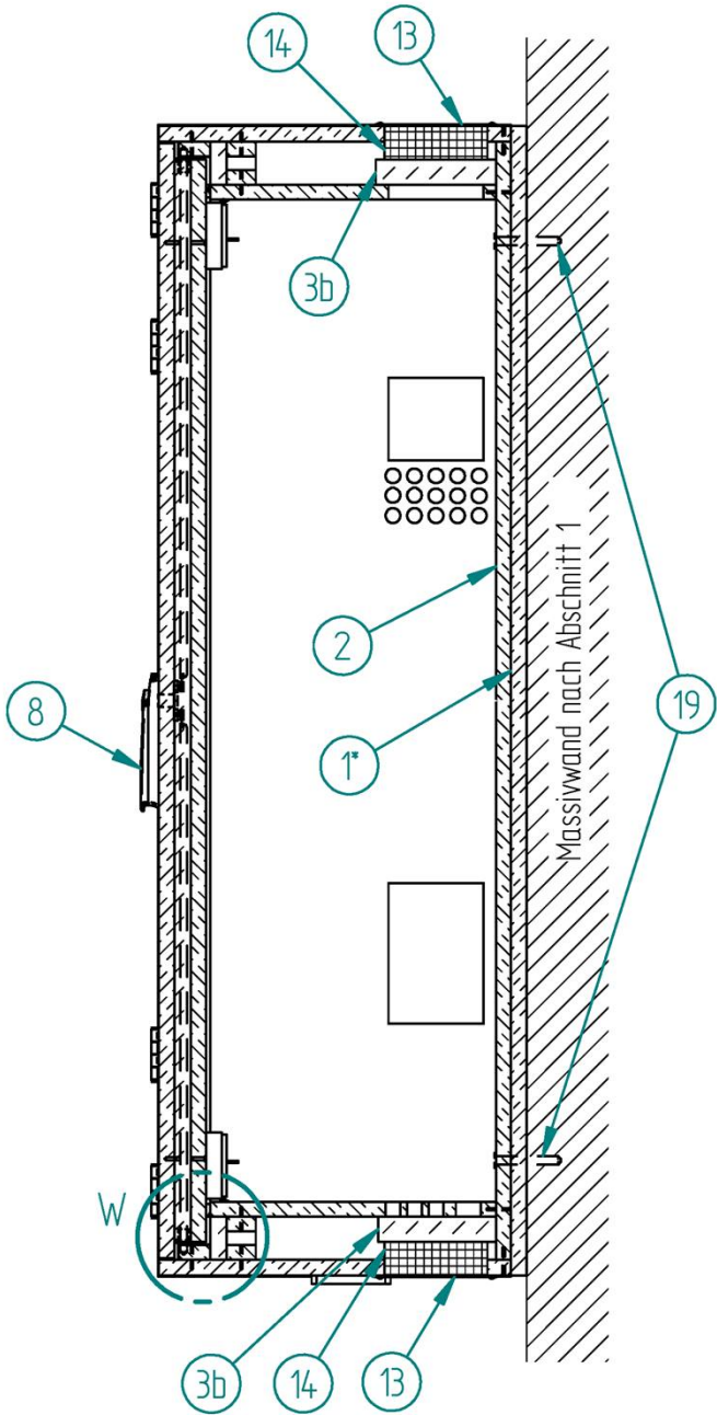
Schnitt D-D
