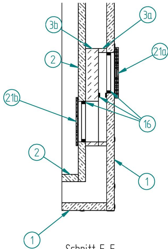
Schnitt F-F
