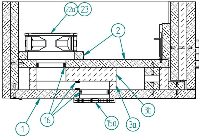
Schnitt E-E
