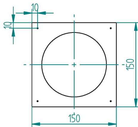
Ansicht von oben ohne Axiallüfter
