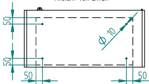
FSE-30 stehend vor leichter Trennwand Ansicht von unten
