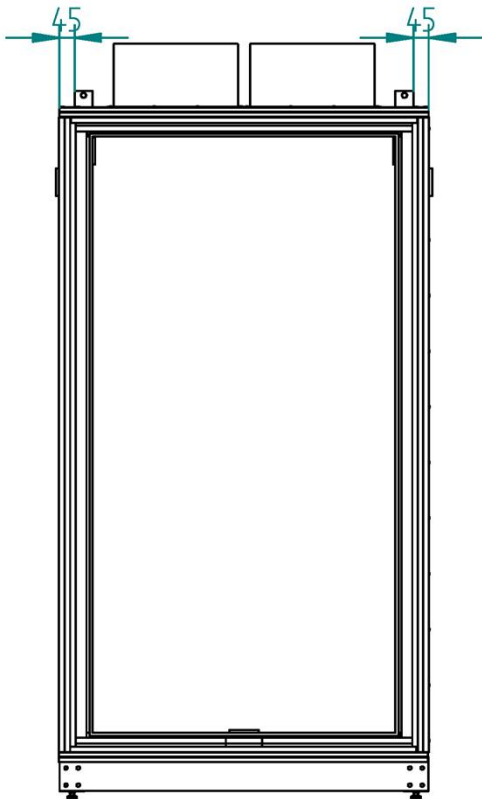
Standgehäuse, wandstehend
