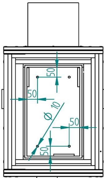
Wandgehäuse
