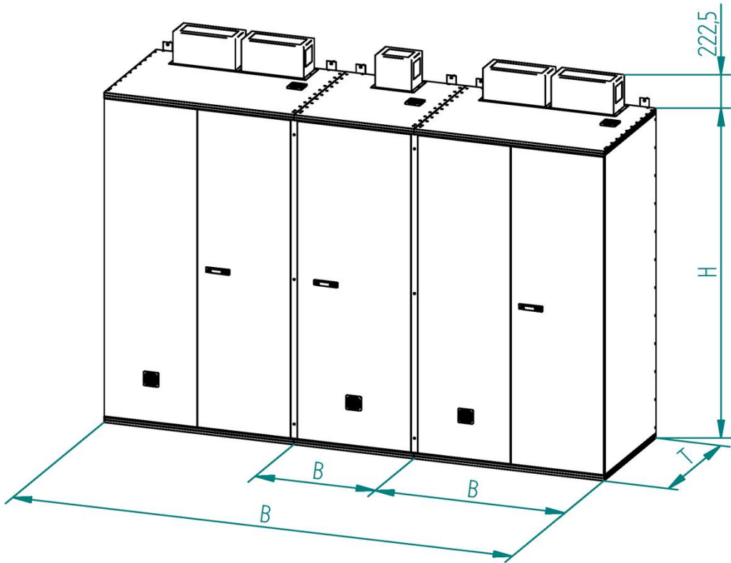
Bsp. Anreihung Typ Violution S-90 multi 2 x zweiflügelige Ausführung 1 x einflügelige Ausführung
