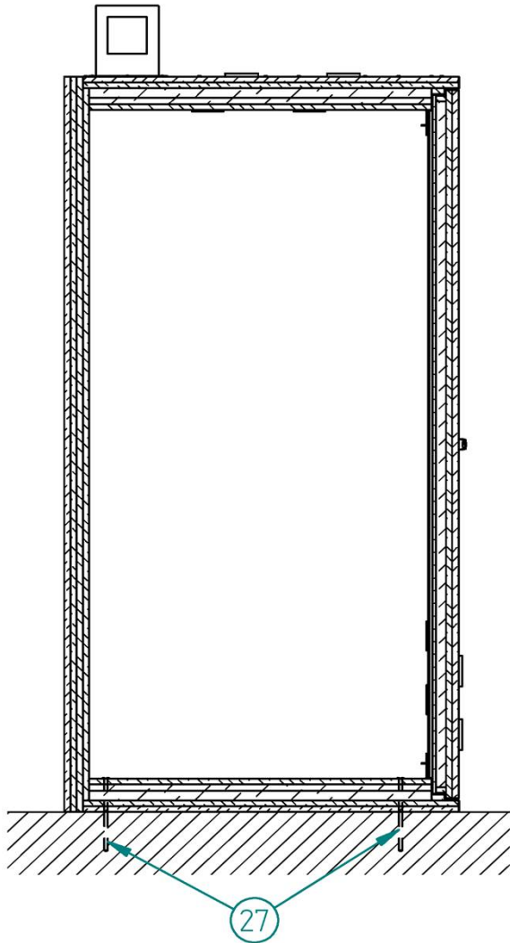
Vertikalschnitt Standgehäuse, freistehend
