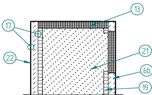
Schnitt J-J
