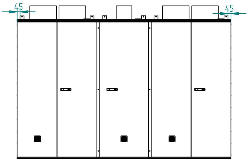
Standgehäuse, in Anreihung
