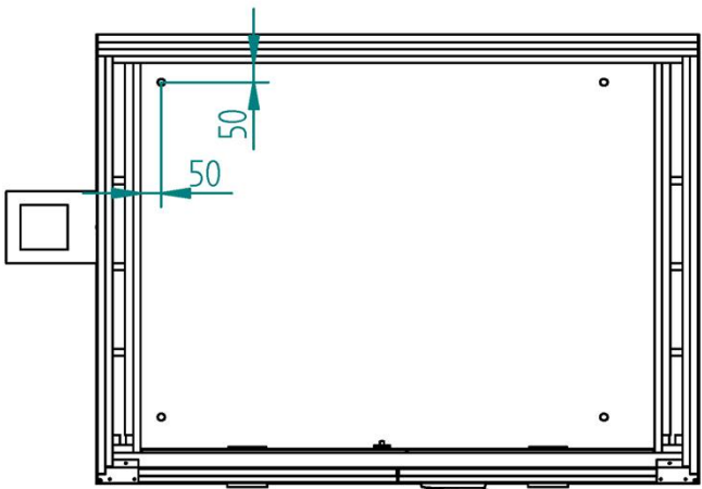
Standgehäuse, freistehend Ansicht von oben ohne Deckel
