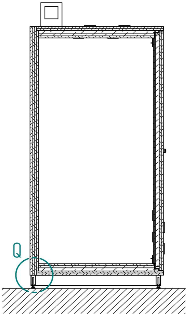
Schnitt K-K
