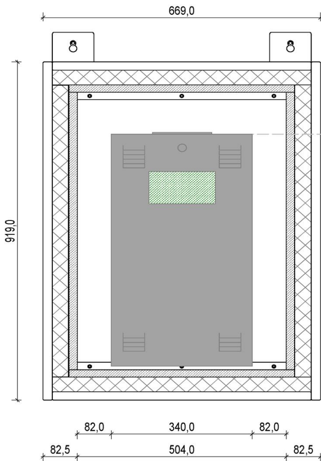
Schnitt A-A
