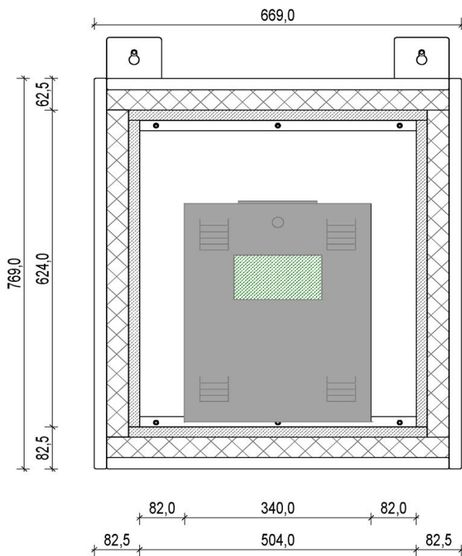
Schnitt C-C
