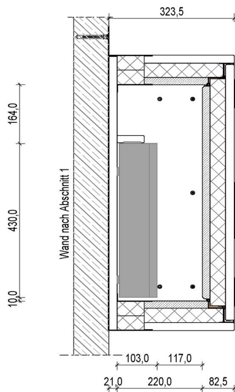
Schnitt D-D
