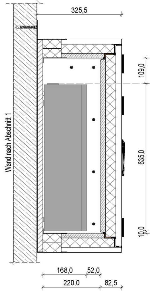
Schnitt B-B
