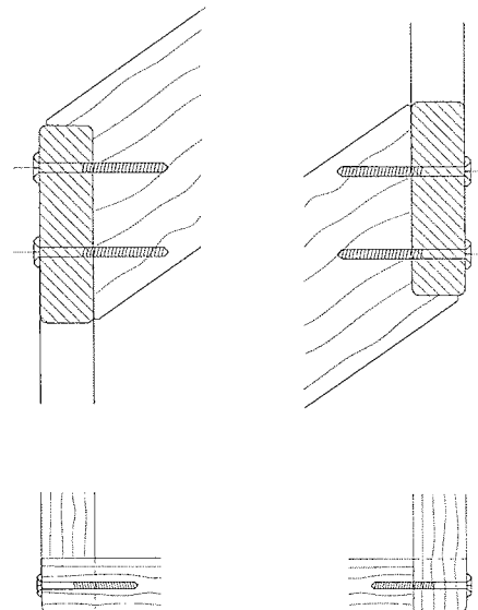
Treppenbauschraube
