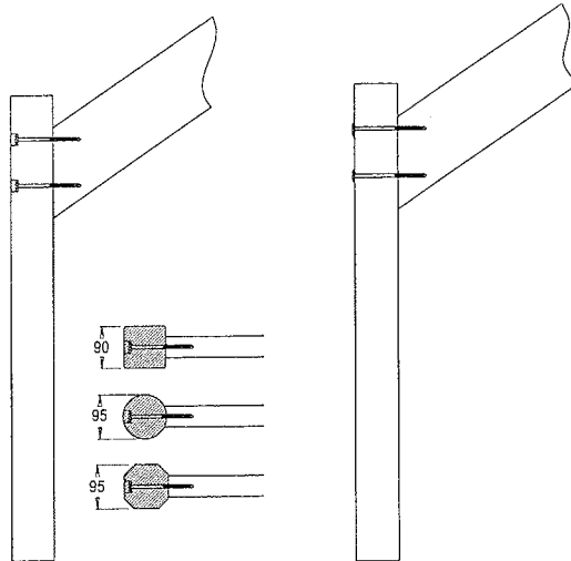
Schraubverbindung
