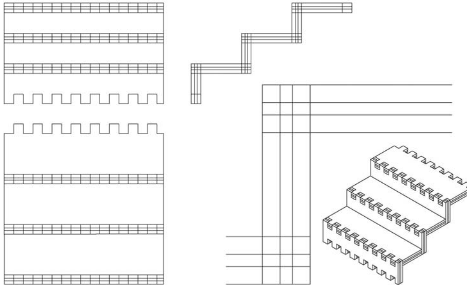
Setzstufe senkrecht
