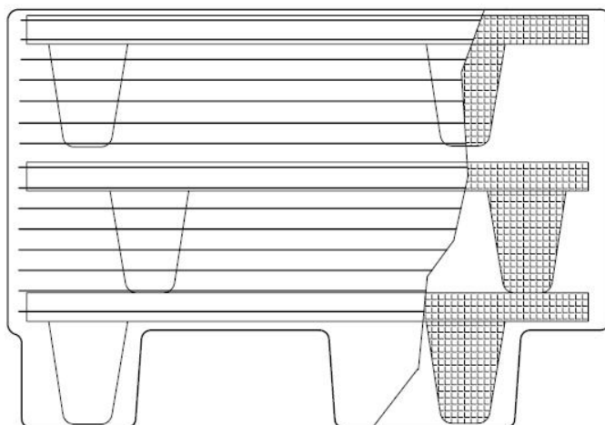
Sicherheitspalette Typ WRP-96 Schnltt mit max. Anzahl Paletten
