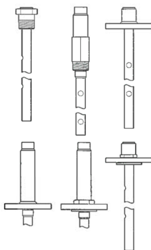
Koaxialsonde 3A, 3B
