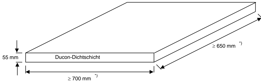
Bild 1: Probekörper
