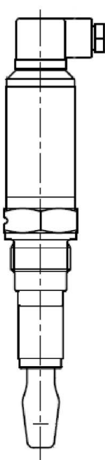
Gewindemontage (Verlängerung)
