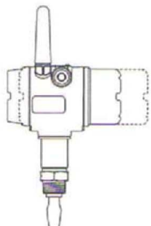
Gewindemontage (Standardlänge)
