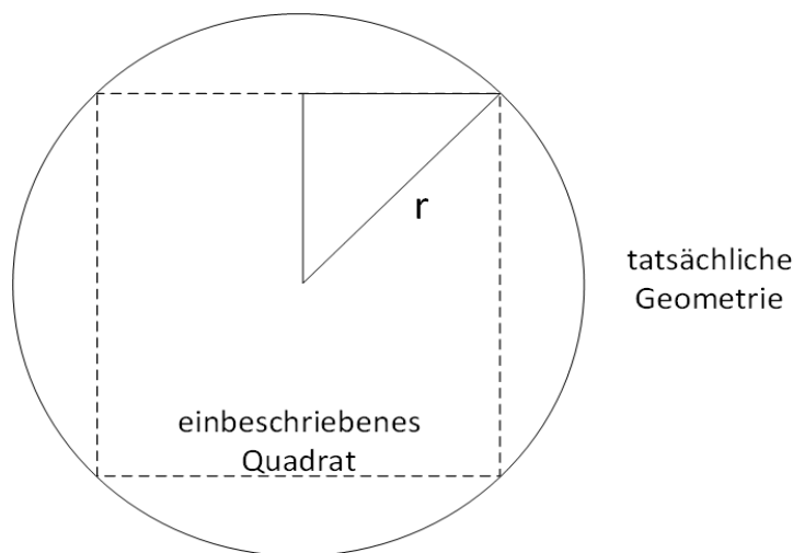
Abbildung 1: Ansatzbare Fläche bei runden Lagern zur Ermittlung des Formfaktors S_{mod}
