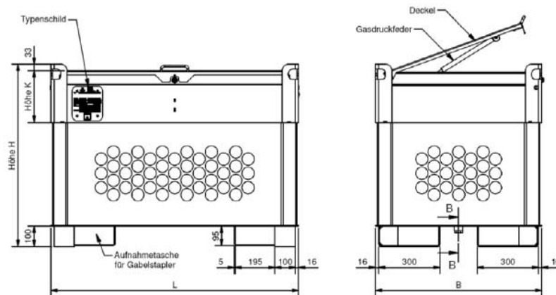
Übersichtszeichnung Typ "KC Quadro C..."
