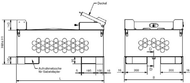
Übersichtszeichnung Typ "KC Quadro C-AG..."
