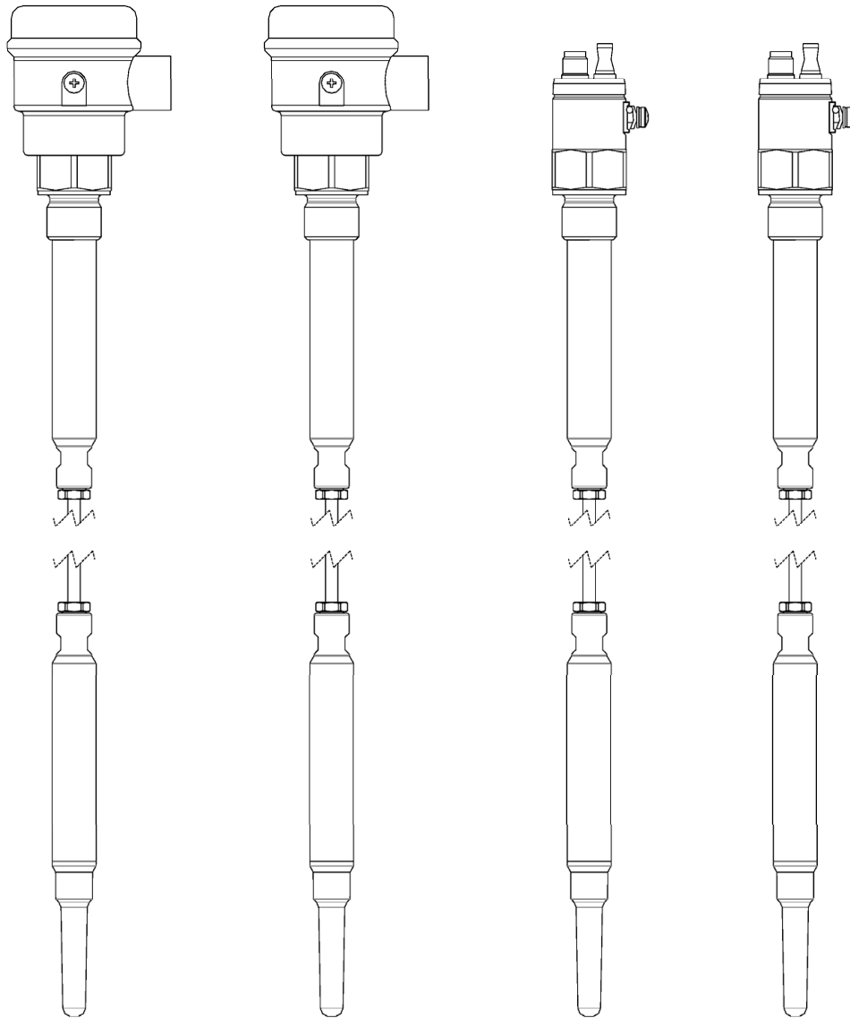
Abb. 3 Version mit Kabelverlängerung Typ CN 7150
