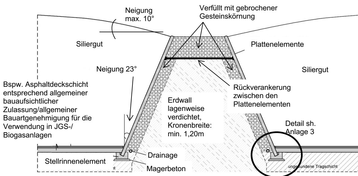
Abbildung 2: Mittelwall – Schnitt
