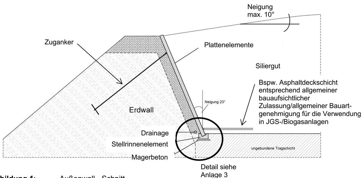
Abbildung 1: Außenwall - Schnitt
