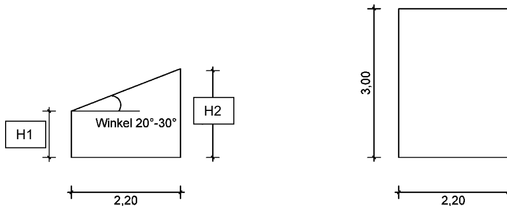
Plattenelement Typ 1
